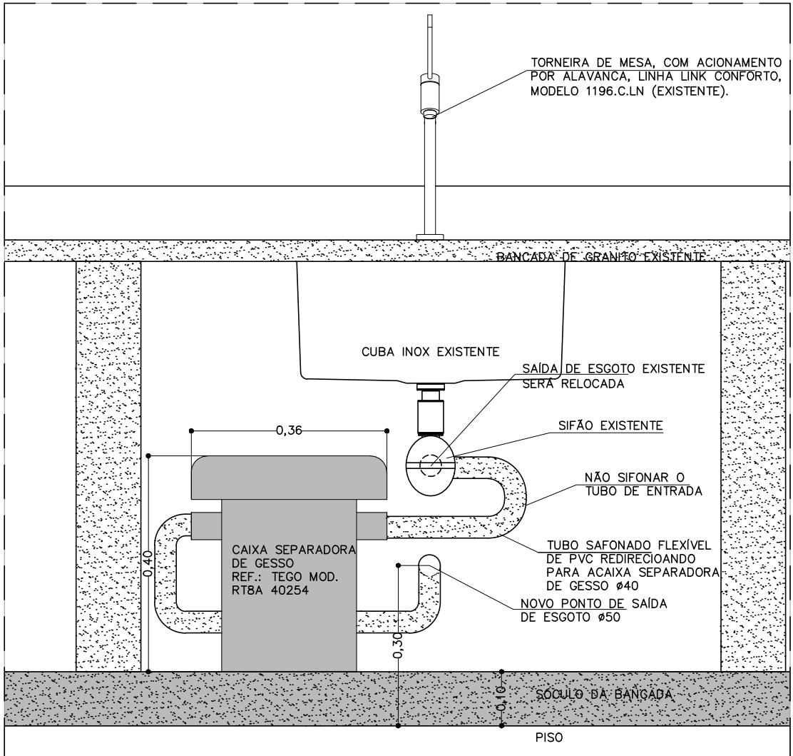
DETALHE DA INSTALAÇÃO DA CAIXA SEPARADORA DE GESSO VISTA FRONTAL ESCALA 1:10
